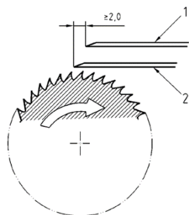
Figura 11 - Detalhe do dispositivo de lâmina dupla
