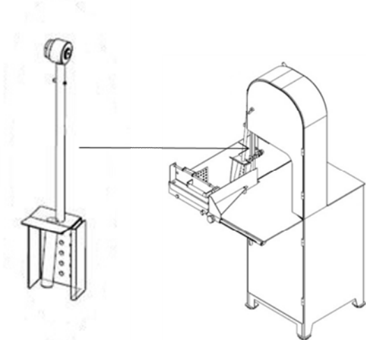
Figura 2 - Exemplo de dispositivo para proteção da mão do trabalhador Fonte: Arquivo da subcomissão de máquinas da CNTT da NR-36
